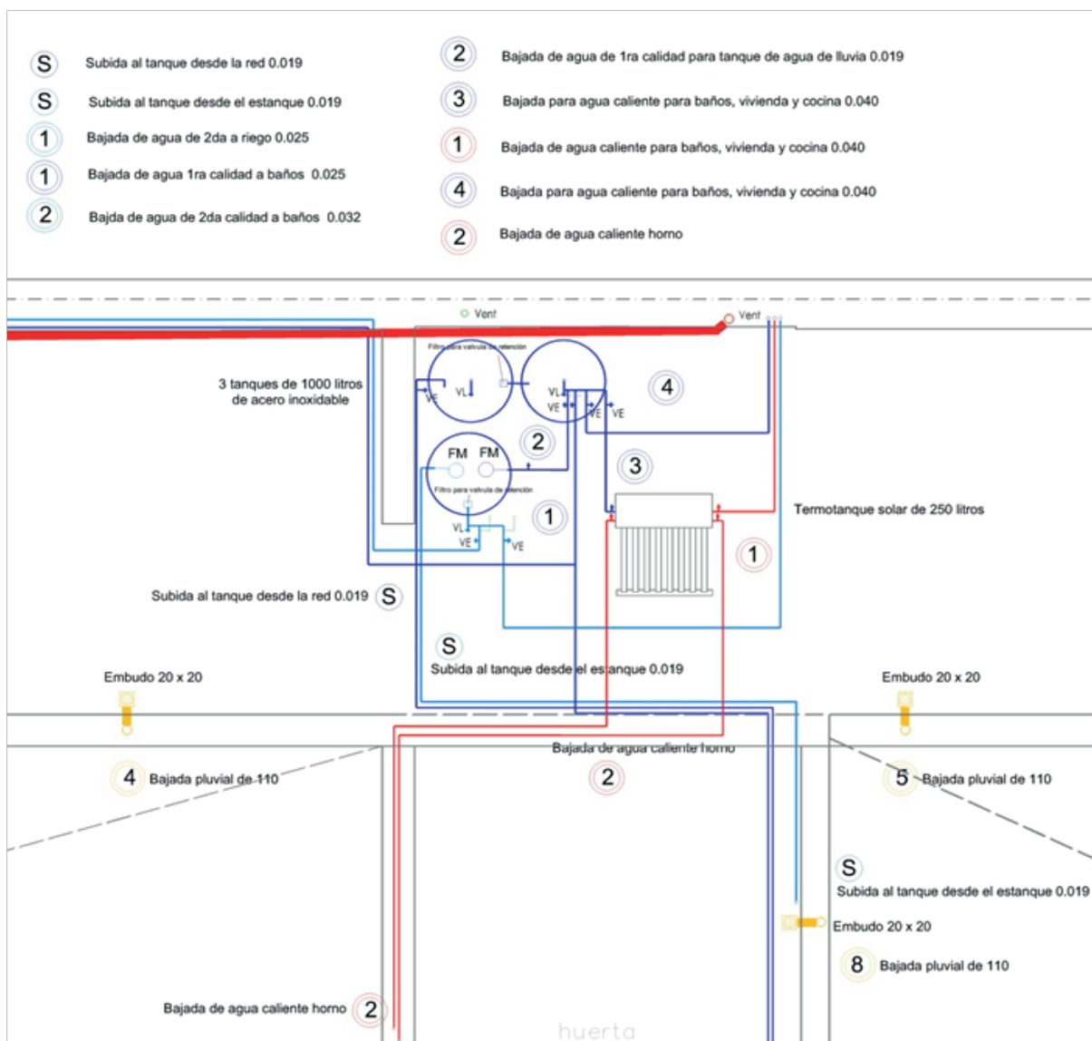
Planta de la instalación en la terraza
